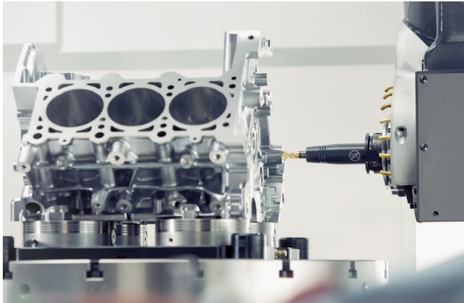
Obrábění hlavy válců s TENDO Slim 4ax
